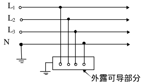
图 4 TT 系统
