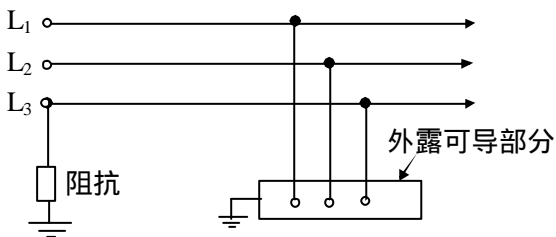
图 5 IT 系统
