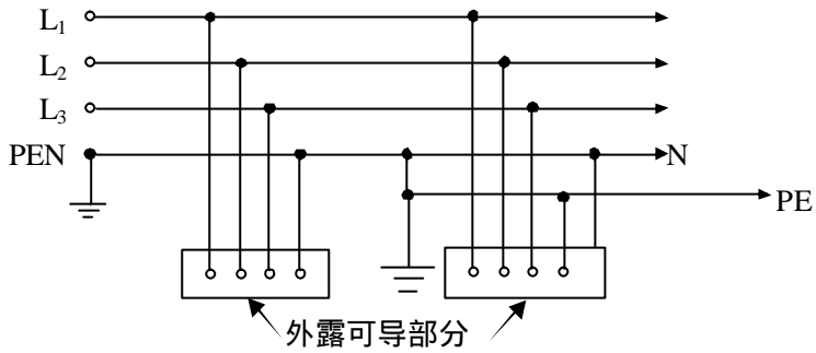
图 2 TN-C-S 系统
