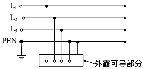
图 3 TN-C 系统
