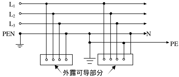
图 2 TN-C-S 系统
