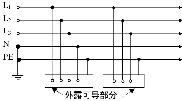
图 1 TN-S 系统
