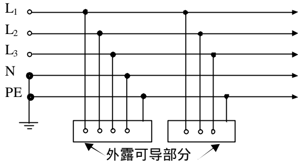
图 1 TN-S 系统
